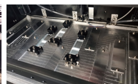
喷头底板 可支持3-16个打印喷头排列，更好的为客户扩展打印空间；
